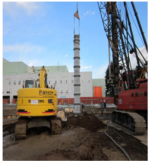
【煙突部の基礎杭建込み】
