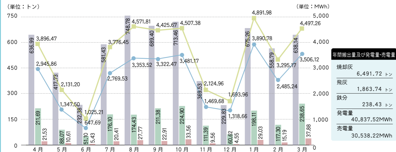
令和2年度 搬出実績及び発電量・売電量
